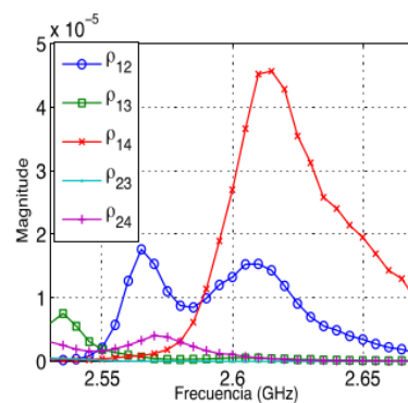
Figura 9. Magnitud de los coeficientes de correlación calculados a través de los parámetros S.
