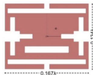
Figura 1. Diseño de la antena tipo patch miniaturizada utilizando slots para operar a 2,6 GHz.
