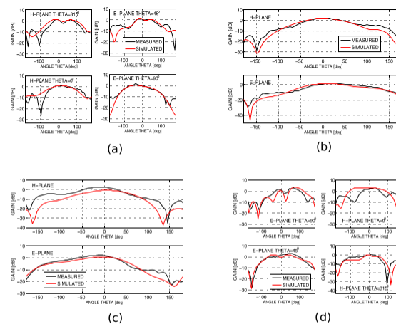
Figura 7. Patrones de radiación en 2D de cada antena medidos (línea negra) y simulados (línea roja). (a) Antena #1. (b) Antena #2. (c) Antena #3. (d) Antena #4. Ganancia dada en dB.
