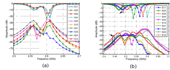
Figura 6. Magnitud de los parámetros S del arreglo propuesto en dB. (a) Simulados. (b) Medidos
