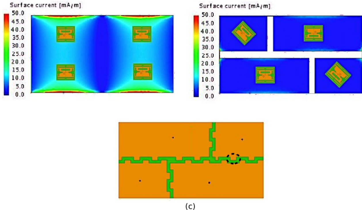
Figura 3. Distribución de corriente total en mA/m, en la frecuencia de 2,6 GHz de (a) plano de tierra de referencia, (b) plano de tierra modificado con slots (sin corrugar), y (c) plano de tierra modificado con los pequeños slots rectangulares.
