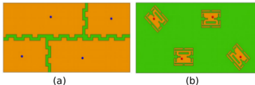
Figura 5. Diseño final del arreglo MIMO. (a) 4-antena sobre el sustrato dieléctrico (PCB). (b) GND modificado con slots corrugados (pequeños triángulos).
