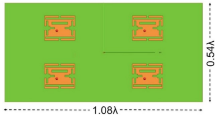
Figura 2. La estructura base o de referencia donde se muestra las cuatro antenas operando a 2,6 GHz.
