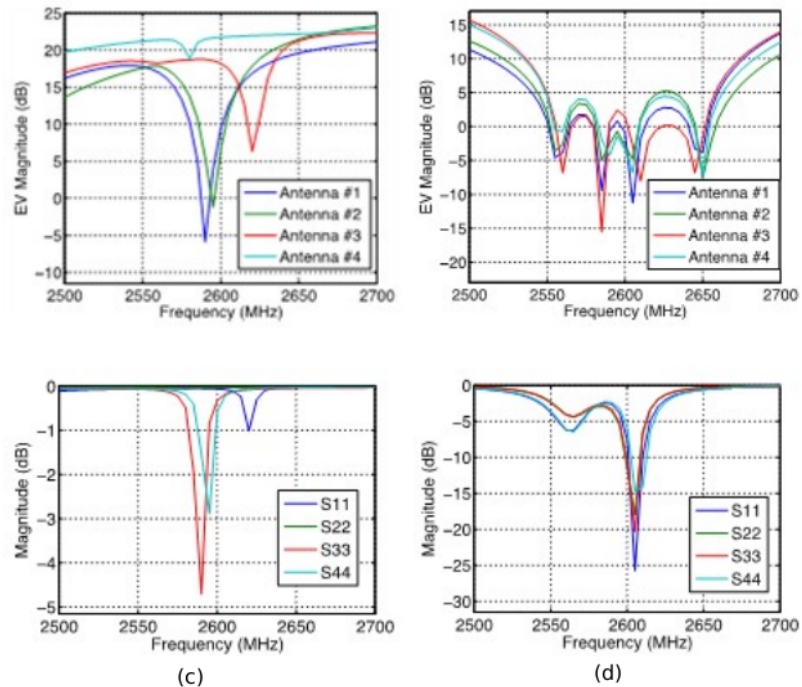
Figura 4. Espectro de eigenvalores NCM del modo dominante de cada antena en dB operando a 2.6 GHz. (a) Eigenvalores antes, y (b) después de aplicar la rotación, (c) pérdidas por retorno (RL) simuladas de cada antena antes, y (d) después de la rotación (ver Fig. 5).
