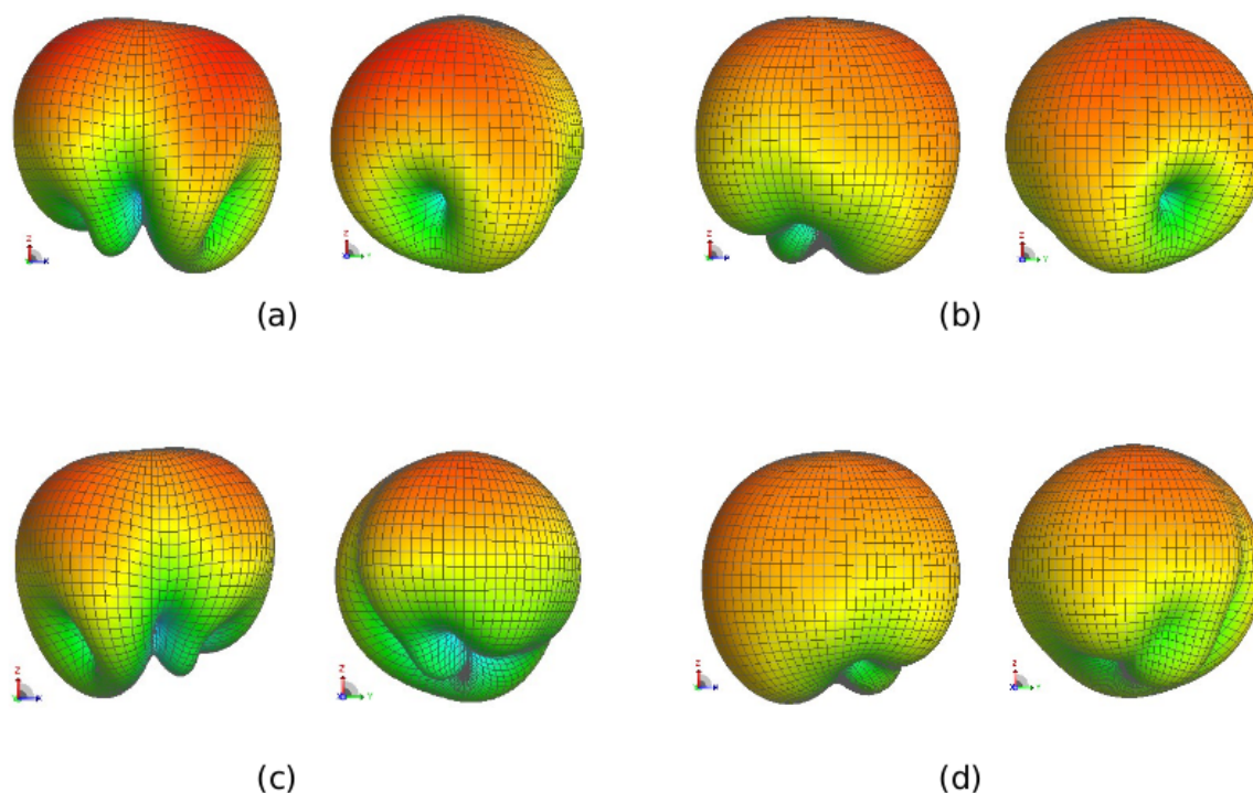
Figura 8. Patrón de radiación simulado en el plano E y en el plano H en 3D de cada antena. (a) Antena #1. (b) Antena #2. (c) Antena #3. (d) Antena #4.
