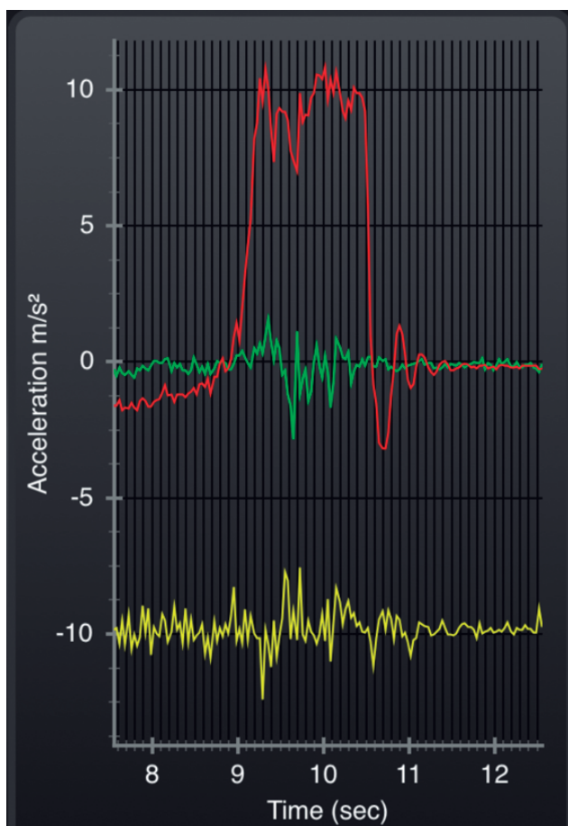
Figura 6. Imagen de los resultados de desaceleración usando un smartphone .
